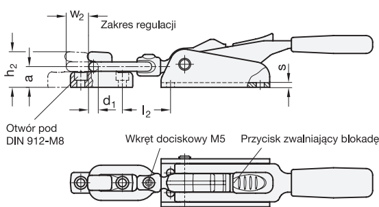
Wymiary montażowe (widok od góry)
