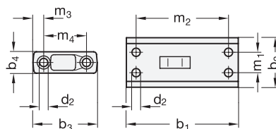
Wymiary montażowe (widok od góry)
